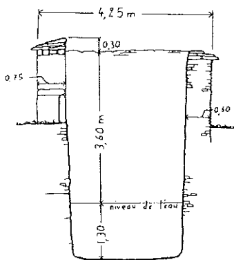
Coupe transversale du puits regardant vers le nord.
