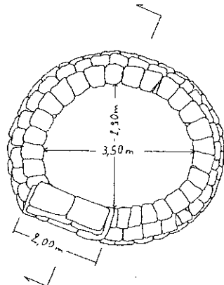
Vue du dessus du puits au niveau de l'arase des murs.
